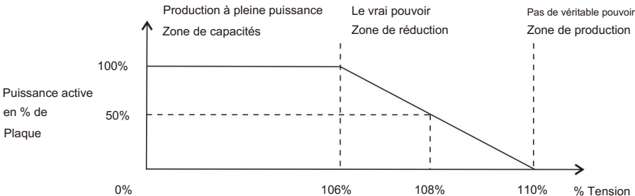
Figure 6.27 Caractéristique Volt-Watt
