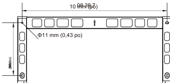
Figure 3.6 Montage mural de l'onduleur
