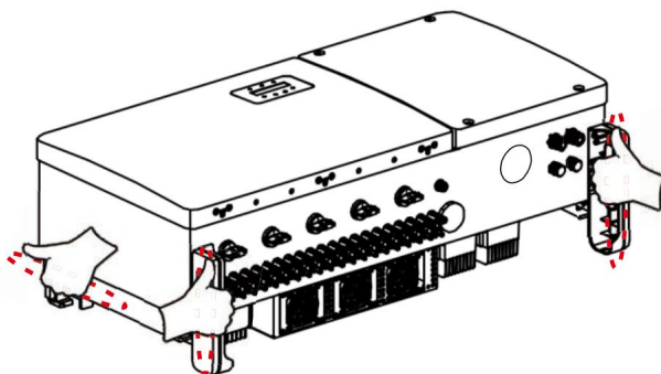
Figure 3.5 Poignées de l'onduleur
