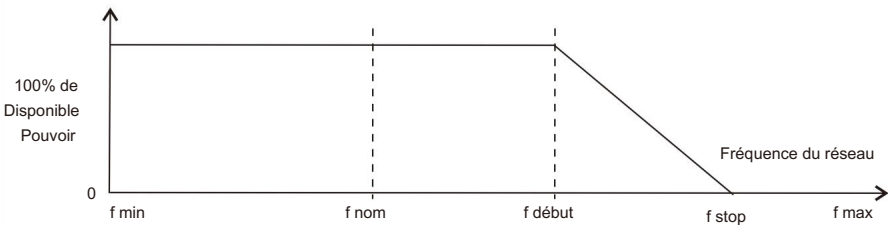
Figure 6.36 Caractéristique Fréquence-Watt
