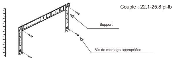
Figure 3.7 Montage mural de l'onduleur
