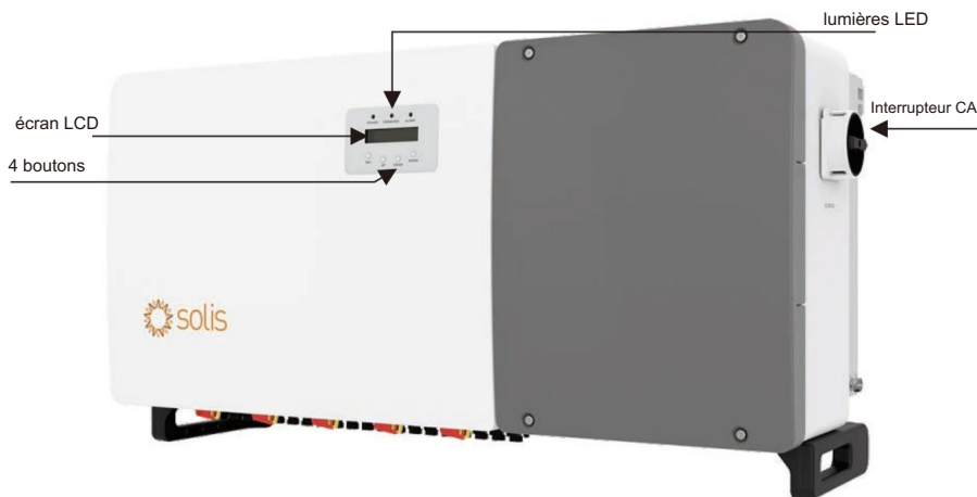
Figure 1.1 Vue de face
