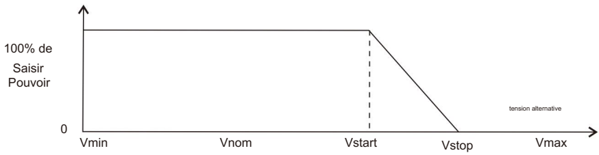
Figure 6.25 Caractéristique Volt-Watt
