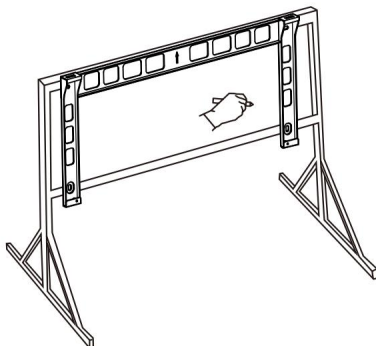
Figure 3.12 Marquer la position du trou
