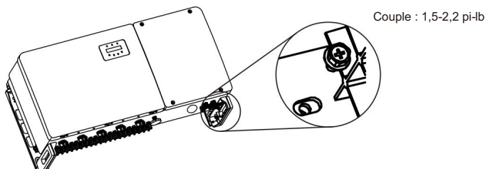
Figure 3.9 Fixer l'onduleur
