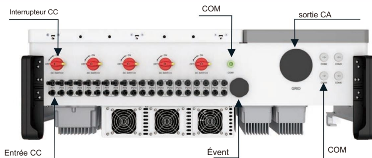
Figure 1.2 Vue de dessous
