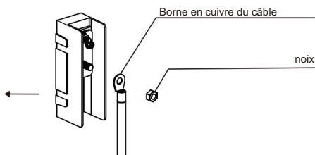
Figure 3.26 Connexion du terminal CA
