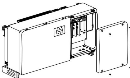
Figure 3.27 Retirez le couvercle de la boîte de jonction
