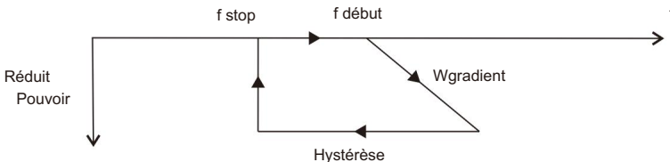
Figure 6.40 Fréquence-Watt (2)
