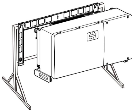
Figure 3.15 Montage de l'onduleur
