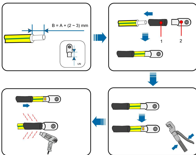
Figure 3.16 Longueur appropriée
