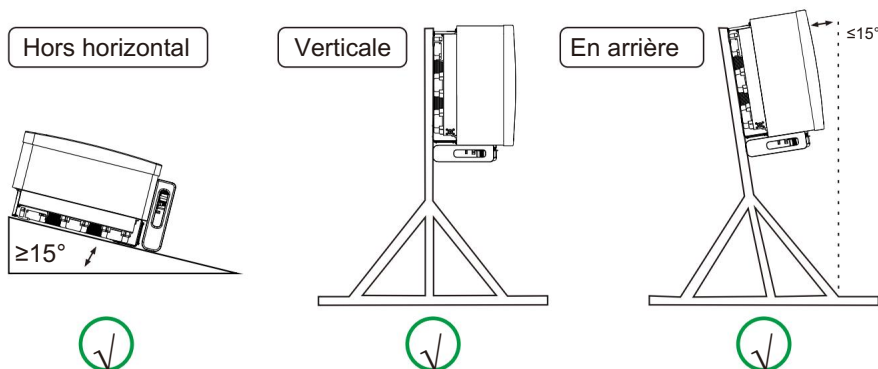
Figure 3.10 Angle d'installation correct
