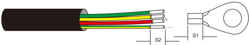
Figure 3.25 Dénudez le câble CA
