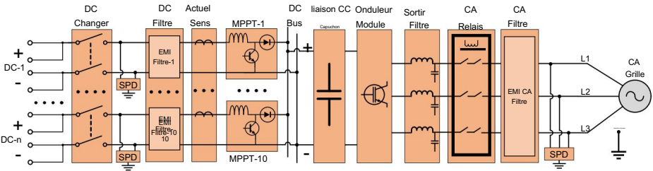
Figure 1.5 Schéma du circuit de l'onduleur
