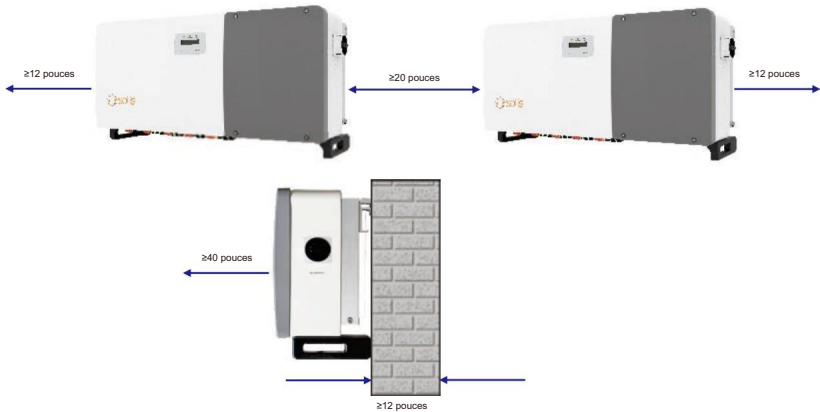
Figure 3.3 Distances respectées entre onduleurs et avec les murs lorsque plusieurs onduleurs sont installés
